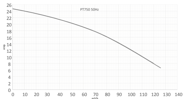
Гидравлич. характеристики
